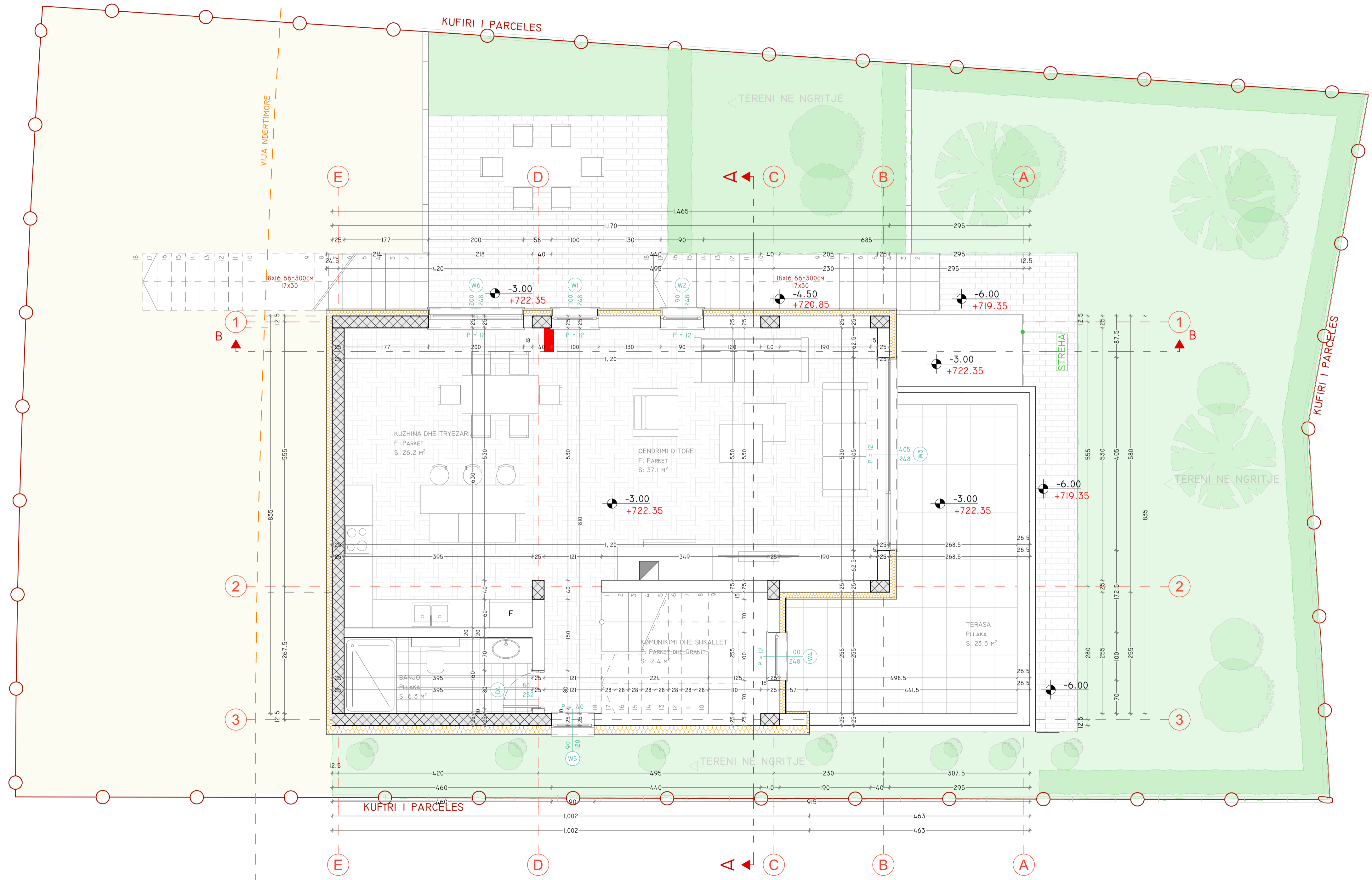
SUTERENI - I SIPERFAQE BRUTO: 121.27m 2
